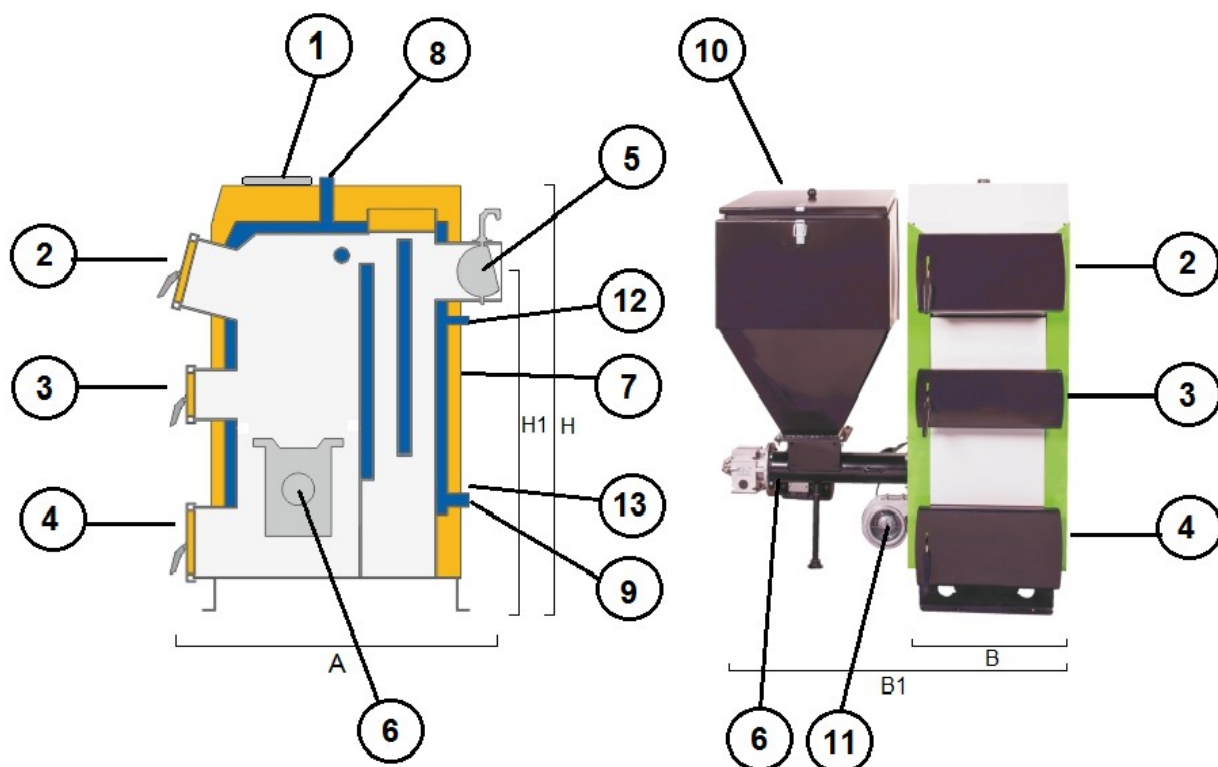
RYS. 1. PRZEKRÓJ KOTŁA V7
